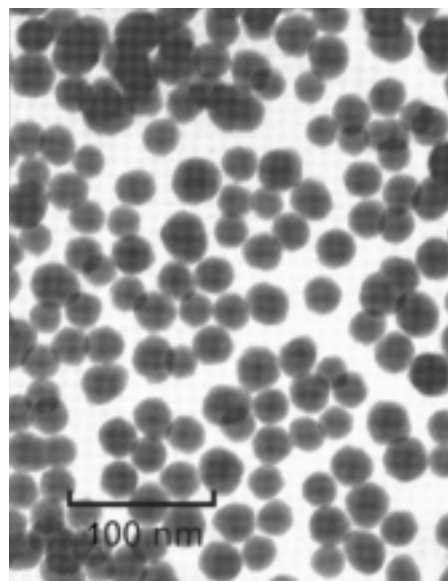
Abb. 1: TEM-Aufnahme eines mit Nano-Partikeln gefüllten Composite Harzes.
