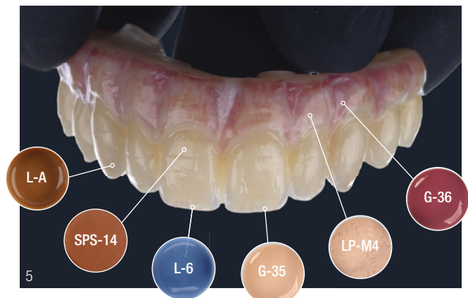
Abb. 4: Im Bereich der Zähne wurde L-NFL (Lustre Neutral Fluor), eine neutrale, stark fluoreszierende Paste, aufgetragen. Sie dient als Verbindungsschicht und verleiht dem Zirkonoxid Fluoreszenz. Im Gingivabereich wurde als Verbindungsschicht L-N (Lustre Neutral) aufgetragen, eine Paste, die keine Fluoreszenz aufweist. – Abb. 5: Mit L-A (Lustre Body A) wurde der gewünschte Farbton erreicht. Mit SPS-14 (Spectrum Stain 14 Deep Orange) wurde das Chroma im Zervikalbereich erhöht. Mit G-35 (Lustre Gum Intensive Cream) wurde der natürliche Halo-Effekt verstärkt. Mit L-6 (Lustre Enamel Effect 6 Dark Blue) wurde ein bläulich-transluzenter Effekt erzielt. Schließlich wurden LP-M4 (Lustre Modifier Brown) und G-36 (Lustre Gum Intensive Red) zur Charakterisierung der erhabenen bzw. vertieften Bereiche des Gingivaanteils verwendet.
