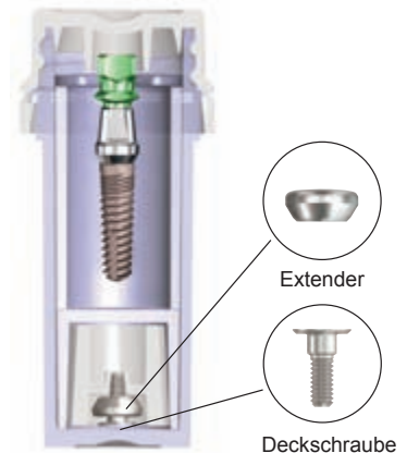
Deckschraube
