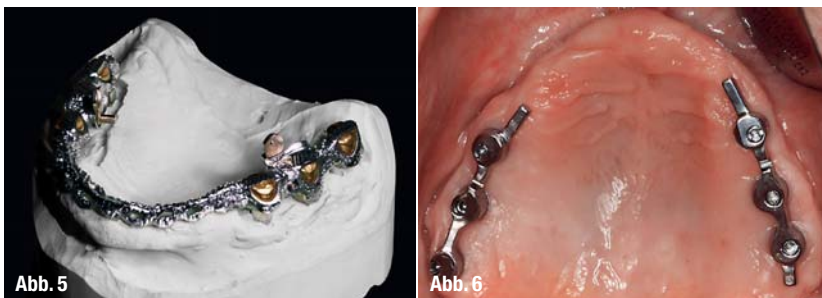
Abb. 5_ Arbeitsmodell mit Stegen, Stegreitern, Tertiärstruktur und eingesetzten Riegeln.
