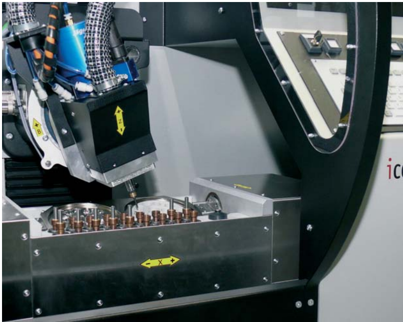
Detailsicht 550i: Hochleistungs-5-Achsmaschine für alle fräsbaaren Dentalwerkstoffe.
