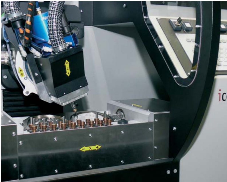
Detailsicht 550i: Hochleistungs-5-Achsmaschine für alle fräsbaren Dentalwerkstoffe.
