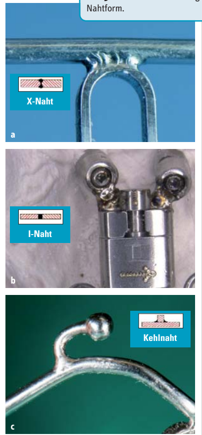
Abb. 3a–c: Schweißverbindungen: Nahtform.
