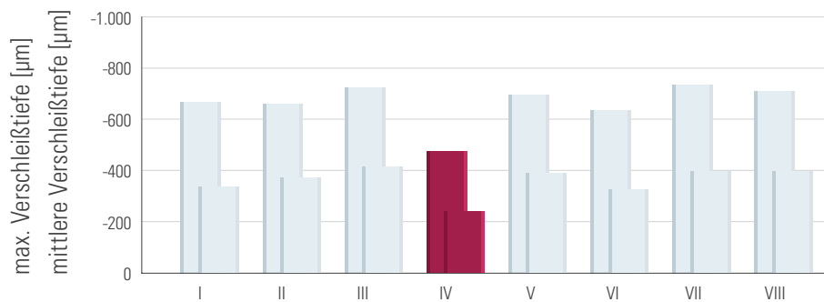
Niedrigste Abrasionswerte bei VITA PHYSIODENS® aus MRP-Material
