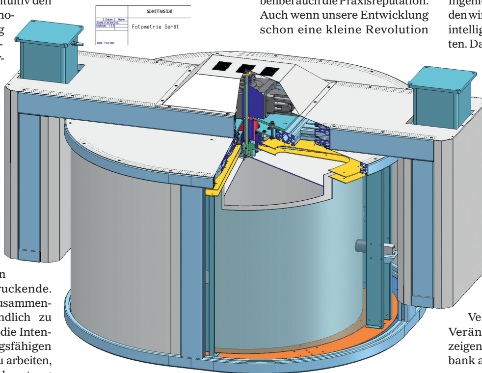
Abb. 6: Technische Zeichnung.
