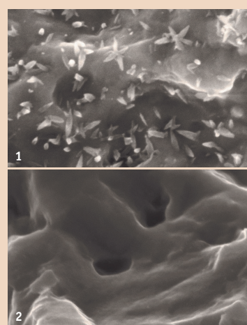
Abb. 1: Nanostrukturen auf SLActive®-Oberfläche. – Abb. 2: SLA®-Oberfläche ohne Nanostrukturen.
