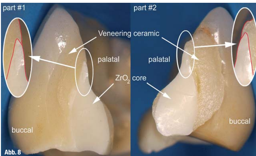
Abb. 8 Fraktur einer verblendeten ZrO 2 -Brücke. Das Gerüst wurde palatinal eingeschliffen (spitz zulaufende Tropfenform) und bot der Verblendung keine ausreichende Unterstützung. Die überdimensionierte Verblendschicht geriet unter Zugspannung. Abb. 9 Chipping-Anteil in der Praxis.
