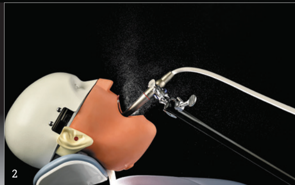
2 Winkelstück mit Sprayluft
