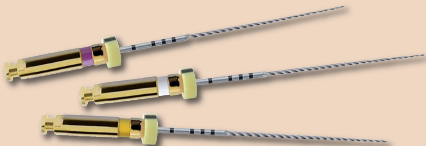
PathFile™ – rotierende NiTi-Instrumente von DENTSPLY Maillefer. PathFile™ Nr. 1 (violett), Spitze ISO 013; PathFile™ Nr. 2 (weiß), Spitze ISO 016; PathFile™ Nr. 3 (gelb), Spitze ISO 019. Konizität 2%. Endomotor: Drehzahl 300 min -1 , Drehmoment 5–6 Ncm.
