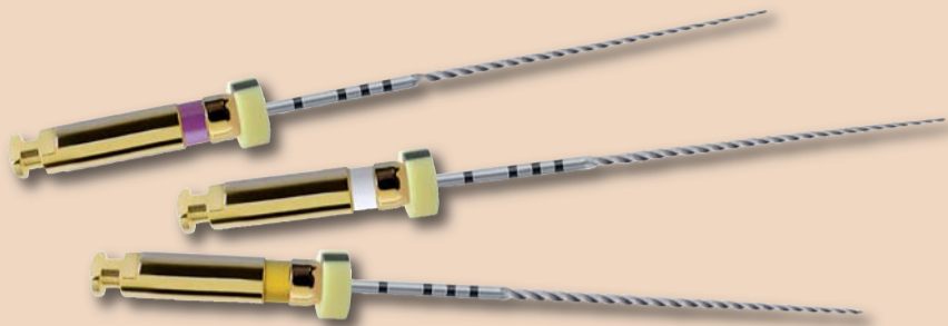
PathFile™ – rotierende NiTi-Instrumente von DENTSPPLY Maillefer. PathFile™ Nr. 1 (violett), Spitze ISO 013; PathFile™ Nr. 2 (weiß), Spitze ISO 016; PathFile™ Nr. 3 (gelb), Spitze ISO 019. Konizität 2%. Endomotor: Drehzahl 300 min -1 , Drehmoment 5–6 Ncm.
