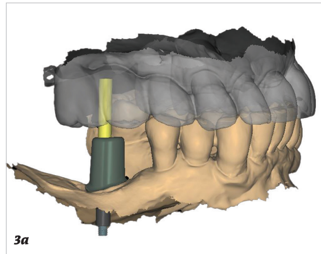
Abb. 3a–d: Digitale Fertigung von implantatgetragenen Zahnersatz: Zusammenführen der Scandaten in der Laborsoftware (a), digitale Konstruktion (b), Einzelzahnrestauration im gedruckten Modell (c), fertiggestellte Hybridabutmentkrone (d).
