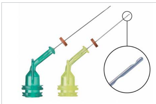
Abb. 6: Der NaviTip Sideport dient als Spülkanüle auch in engsten Kanälen; seitlicher Flüssigkeitsaustritt verhindert Transport über den Apex hinaus.
