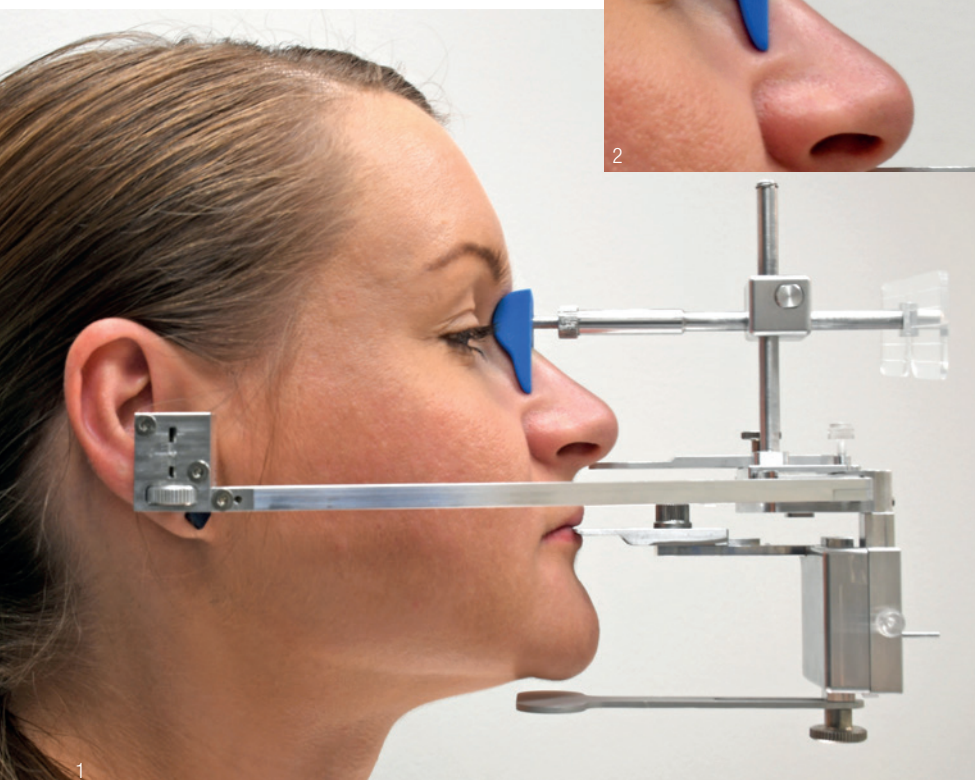
Abb. 1: therafaceline – das neue Gesichtsbogensystem in situ. Abb. 2: Ansicht der Nasenstütze inklusive des Bipupillarlineals. Die Nasenstütze kann zudem vertikal nach der Camperschen Ebene und der Patientenhorizontalen ausgerichtet werden.
