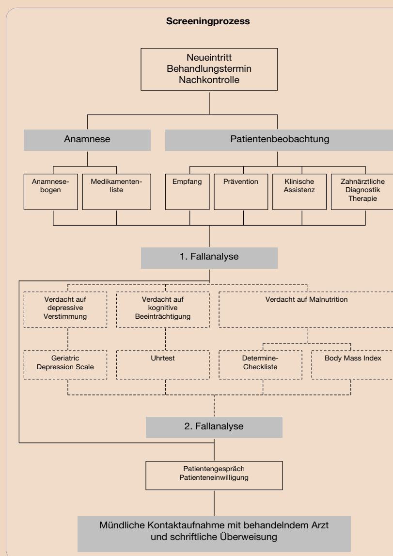
Abb. 2: Screeningprozess.
