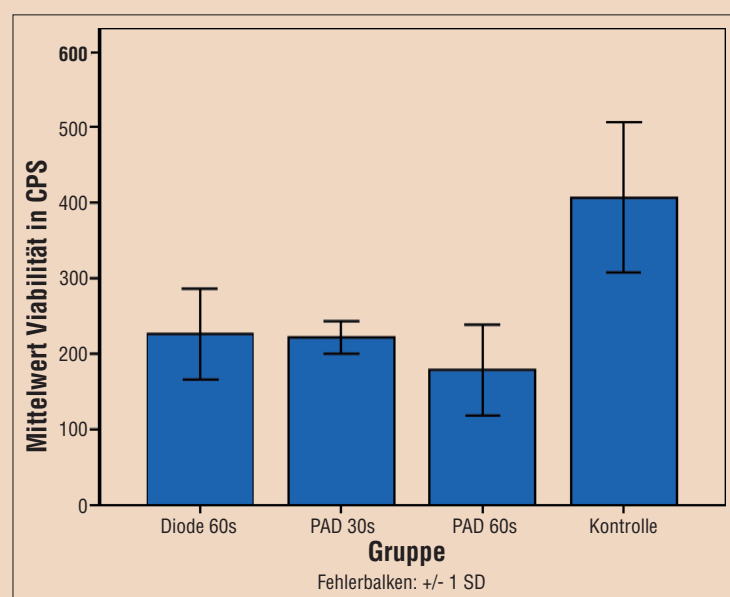
Abb. 3: Übersicht über die Viabilitäten in den Biofilmen gemessen in Counts Per Second (CPS) – nativ sowie nach den Behandlungsprozeduren.
