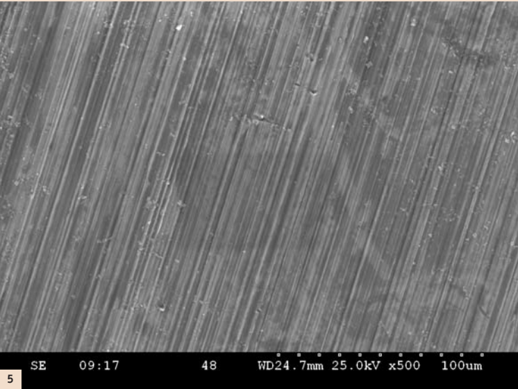
Abb. 3: Rasterelektronenmikroskopische Aufnahme einer säuregeätzten und gestrahlten Titanoberfläche (Promote®, CAMLOG Vertriebs GmbH, Wimsheim, Deutschland) in 500-facher Vergrösserung. – Abb. 4: Rasterelektronenmikroskopische Aufnahme nach Behandlung einer Promote®-Oberfläche mit der Hans K Titan-Reinigungsbürste (HK RB-Line 5, Kentzler-Kaschner Dental GmbH, Ellwangen, Deutschland) in 500-facher Vergrösserung. Die Makro- und Mikroporositäten werden in eine glatte Oberfläche überführt, die ähnlich einer maschinellen Titanimplantatoberfläche erscheint. – Abb. 5: Rasterelektronenmikroskopische Aufnahme einer industriell gefertigten, maschinellen Titanoberfläche in 500-facher Vergrösserung. Charakteristisch sind die feinen, parallel verlaufenden Rillen. – Abb. 6: CAMLOG-Implantat im Kunststoffkiefer bei Simulation einer periimplantären Defektsituation. Der untere Anteil zeigt die unbehandelte Promote®-Oberfläche, die sich grau und matt darstellt. Der obere Anteil des Implantates wurde bereits mit der Hans K RB-Line 5-Bürste bearbeitet. Die Oberfläche erscheint nach Bürstung deutlich glänzender.
