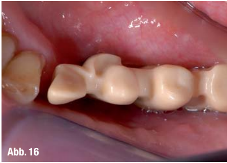
Abb. 16_ CAD/CAM-gefrästes Zirkonbrückengerüst.
