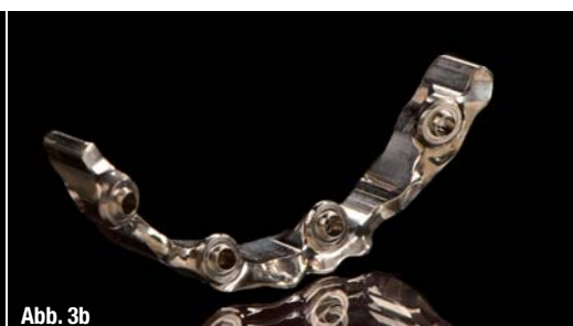
Abb. 3a–c CAD/CAM-generierte Titanstege (Procera ImplantBridge Titanium, Nobel Biocare) zur Stabilisierung herausnehmbarer Restaurationen bieten vor allem bei stark atrophierten Kieferkammern Vorteile in Bezug auf Hygienefähigkeit, Unterstützung der perioralen Muskulatur und Phonetik. CAD-Objekt eines gescannten Steges (a) und der industriell gefertigte Steg auf Implantatniveau (b) garantiert maximale Materialhomogenität und Präzision bei deutlich reduzierten Kosten gegenüber gegossenen Edelmetallkonstruktionen (b und c).
