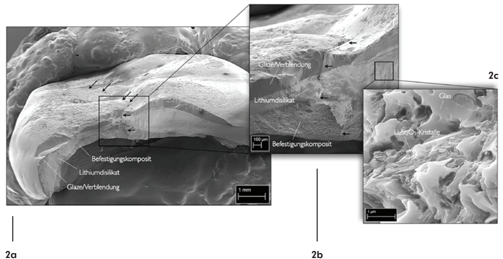
Abb. 2a–c: Rasterelektronenmikroskopische Aufnahmen von der Bruchfläche des Kronenfragments a) in der Übersicht, in Detailaufnahme b) im Bereich des Rissursprungs und c) aus mikroskopischer, kristallografischer Ebene.
