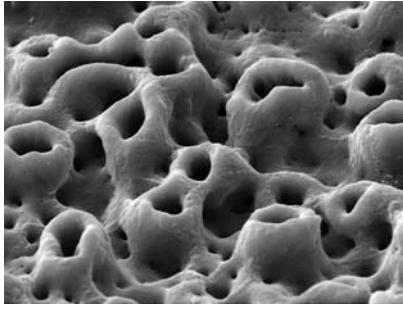
Abb. 2: SEM-Aufnahme der Poren auf der TiUnite®-Oberfläche. – Abb. 3: Präosteoplast auf der TiUnite®-Oberfläche. – Abb. 4: Verankerung des Präosteoplasten über Pseudopodie in einer offenen Pore.
