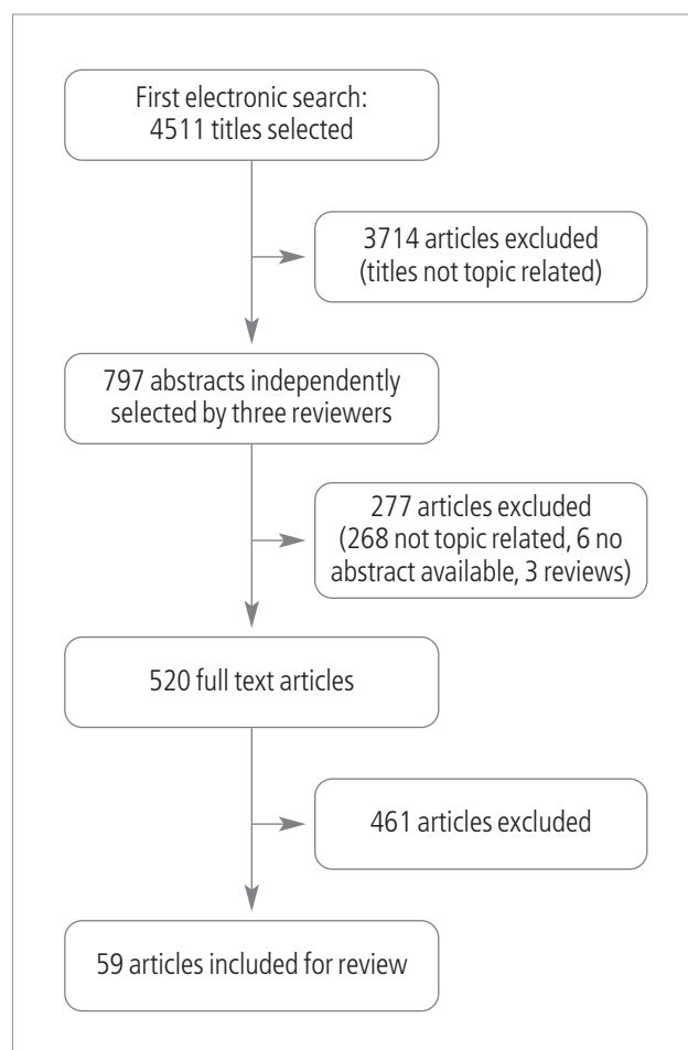
Abb. 1: Artikelauswahl.
