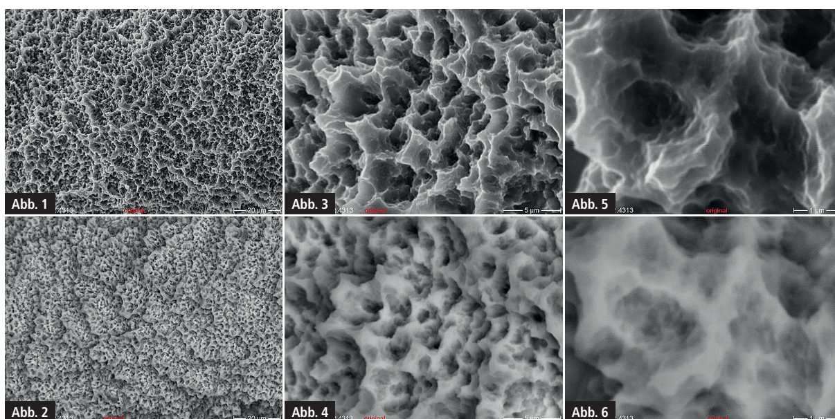
Originale Implantatoberfläche, an einer Gewindespitze —Abb. 1: 1.000:1, SE-Bild.—Abb. 2: 1.000:1, RE-Bild.—Abb. 3: 5.000:1, SE-Bild.—Abb. 4: 5.000:1, RE-Bild.—Abb. 5: 20.000:1, SE-Bild.—Abb. 6: 20.000:1, RE-Bild.
