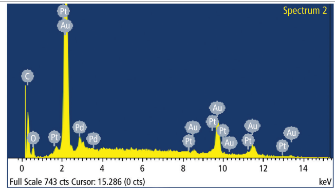
Abb. 11: SEM-EDS-Analyse (Patientenfall: Nachweis von Gold, Platin und Palladium in der Gewebeprobe bei vorausgegangener jahrelanger VMK-Brückenversorgung).
