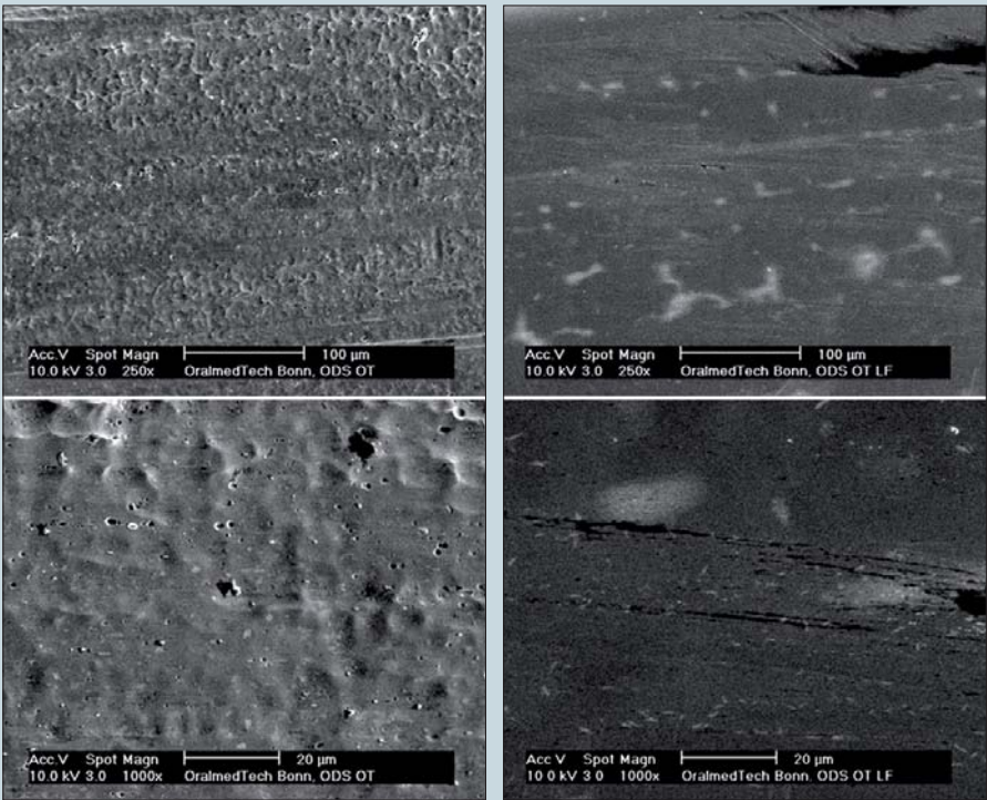
Abb. 9a: Oberflächenbeschaffenheit des unbehandelten Euro NiTi (links) und des vergüteten Euro NiTi LF (rechts).
