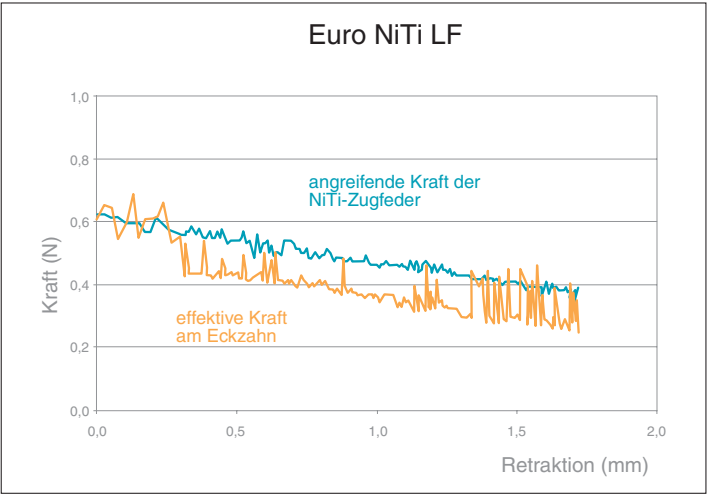
Abb. 4: Beim vergüteten Draht ist die Differenz zwischen blauer und orange Kurve deutlich geringer. Die Friktion konnte signifikant reduziert werden.
