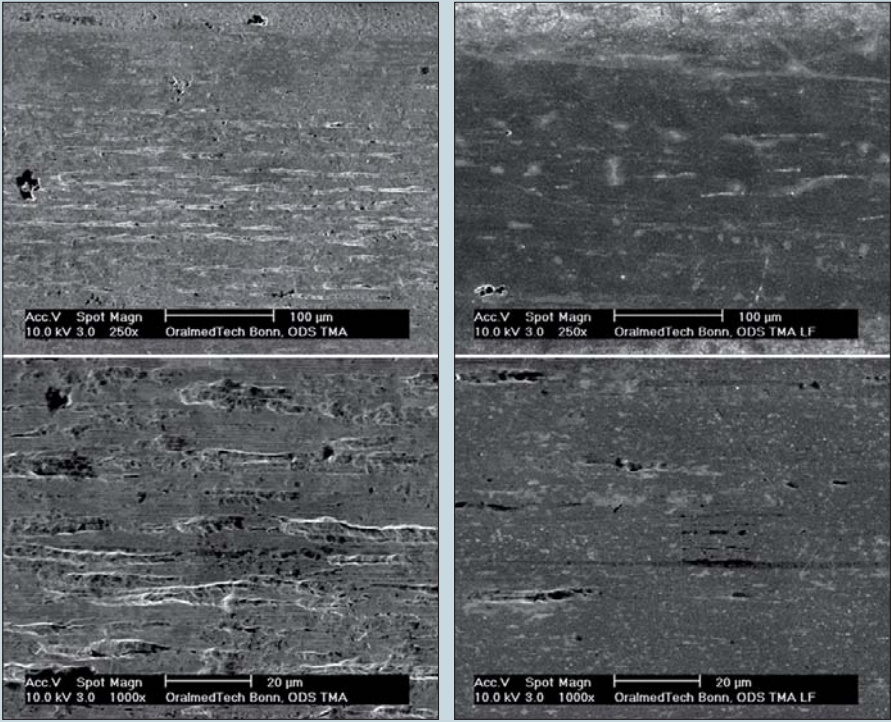
Abb. 9c: Oberflächen des unvergüteten \beta -Titan-Drahtes (links) und oberflächenveredelten \beta -Titan LF (rechts).
