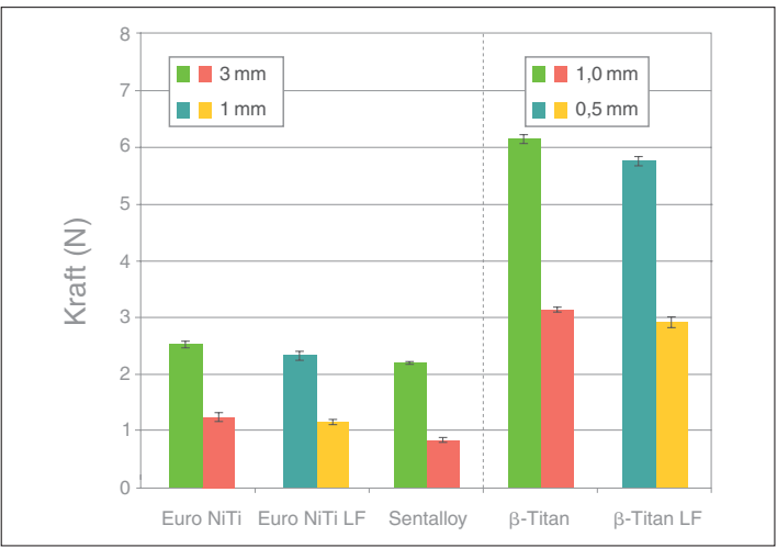
Abb. 6: Geometrieänderungen durch die Oberflächenveredelung: Keine signifikante Veränderung der Abmessungen, alle Bögen innerhalb der vorgegebenen Toleranzen.
