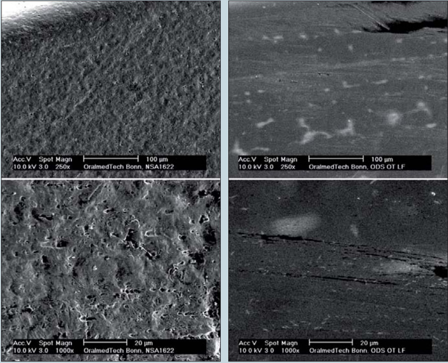
Abb. 9b: Vergleich der Oberflächen des Sentalloy Ion Guard (links) und des Euro NiTi LF (rechts).
