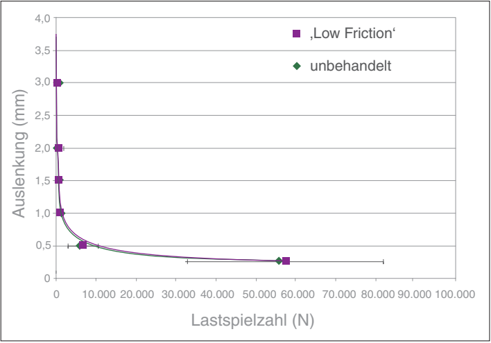
Abb. 8: Wöhlerkurven der beiden behandelten und unvergüteten \beta -Titan-Drähte.
