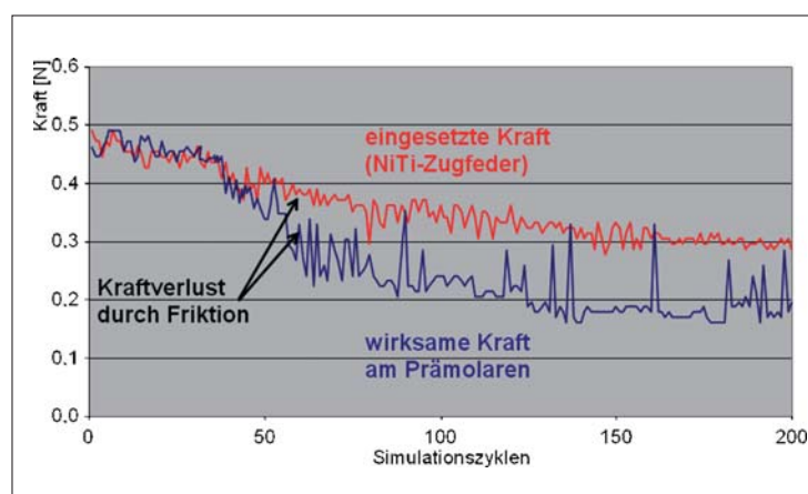
Abb. 5: Darstellung der gemessenen Kräfte der NiTi-Zugfeder und am Prämolarenbracket am Beispiel der Kombination Incognito/16 x 22-Stahldraht. Die Friktion ergibt sich aus der Differenz der beiden Werte (Pfeile). Zu Beginn der Bewegung gleitet das Bracket konfliktfrei am Bogen entlang, daher setzt die Friktion erst nach einer bestimmten Retraktionsstrecke ein, wenn Bracketslot und Führungsbogen in Kontakt kommen.
