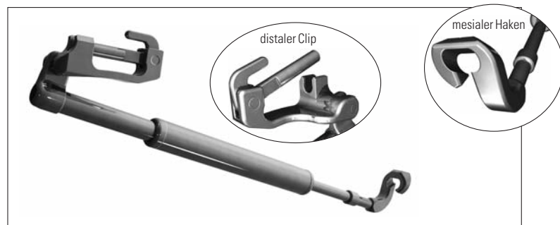
Esprit™ Klasse II-Apparatur.
