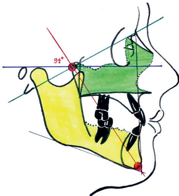
Abb. 5: Lageverhältnis der beiden Kiefer im Kreuz der „Facial Axis“. Der hinterste oberste Punkt der Maxilla und der vorderste unterste Punkt der Mandibula liegen genau auf der Achsolinie und bilden ein 90°-Winkelverhältnis.
