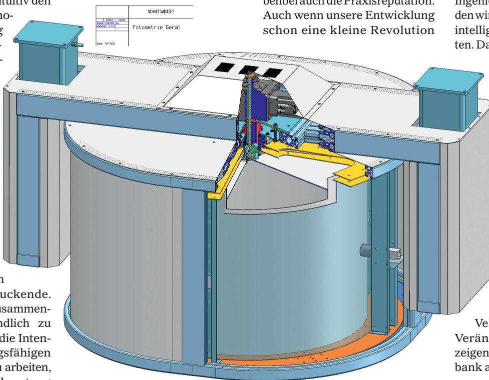
Abb. 6: Technische Zeichnung.
