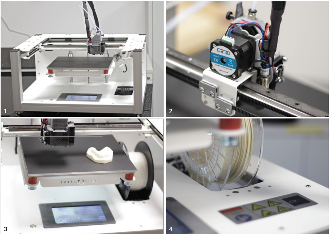
Abb. 1–4: Der OrthoCube® ist an die Bedürfnisse von KFO-Praxen angepasst und setzt auf Filament als Druckmaterial. Abb. 5 und 6: Die optionale Glasvitrine wird in verschiedenfarbigen Gehäusen geliefert (je nach Praxis-CI); die Fotos zeigen die Aufstellung im Eingangs- bereich sowie Wartezimmer. (Fotos 1–6: © Dr. Kai Hinz-Vahle)
