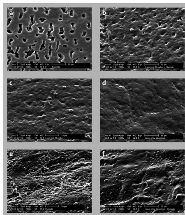
Abb. 4: Übersicht über die detektierten Oberflächenveränderungen in der Rasterelektronenmikroskopie ( 2.000\times, 40^\circ ).
