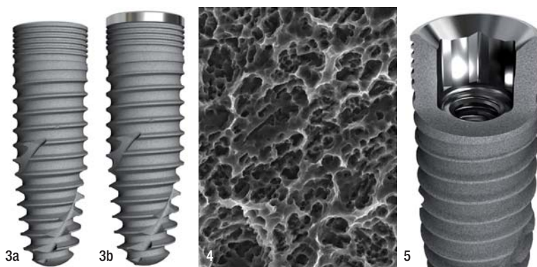
Abb. 3a und b: Neue BEGO Semados® RS- und RSX-Implantatlinien mit Mikrorillenstruktur im Implantathalsbereich. – Abb. 4: Hochreine, homogene, gestrahlte-geätzte TiPurePlus-Oberfläche; gleiche Oberfläche wie S- und RI-Implantate. – Abb. 5: Bewährte konische Innenverbindung: mit 45° mittlerem Konuswinkel und Rotationssicherung durch Innensechskant sowie integriertes Platform-Switching.
