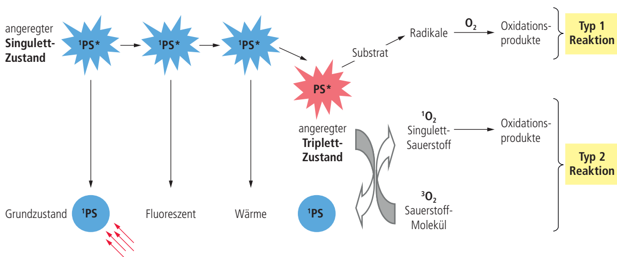
Abb. 1: Fällt auf den Photosensibilizer (PS) Licht einer bestimmten Wellenlänge, wird er zum Singulett-Zustand aktiviert. Dieses instabile Molekül kann durch Energieverlust wieder in den stabilen Zustand oder in einen langlebigeren Triplett-Zustand übergehen. (Grafik nach Soukos & Goodson 6 , modifiziert durch Gonzales & Kross 7 .)
