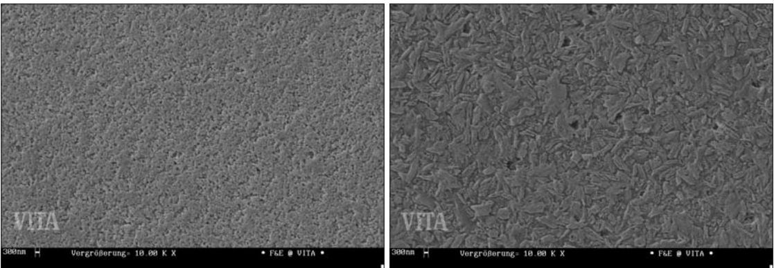
Abb. links: VITA SUPRINITY, REM-Aufnahme, 10.000 x. – Abb. rechts: Lithiumdisilikat, REM-Aufnahme, 10.000 x. – REM-Aufnahmen der glaskeramischen Materialstrukturen. (Quelle: Tech.-Wiss. Doku. VITA SUPRINITY; VITA F&E).
