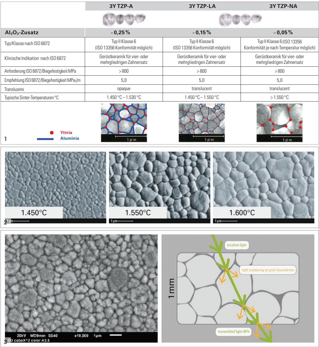
Abb. 1: 3Y-TZP-Typen, unterschieden nach Al 2 O 3 -Anteil. Abb. 2: Effekt des Kornwachstums (3Y-TZP-NA) REM-Aufnahmen (geschliffen und thermisch geätzt). Abb. 3: 5Y-TZP – hybrides Mikrogefüge. REM-Aufnahme (geschliffen und thermisch geätzt).
